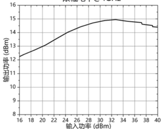
限幅电平@4GHz
