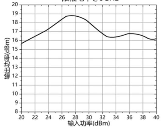
限幅电平@9GHz
